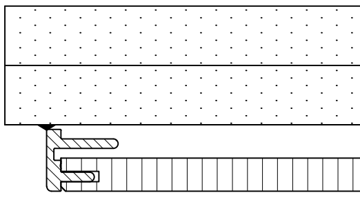
seitlicher Anschluss
