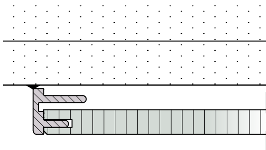
Seitlicher Abschluss Profil A25
