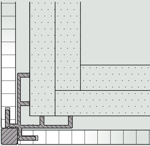
Vierkantprofil
