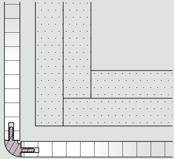
Alu-Viertelstab 90°
